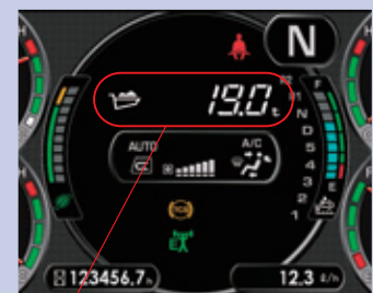
Payload display
